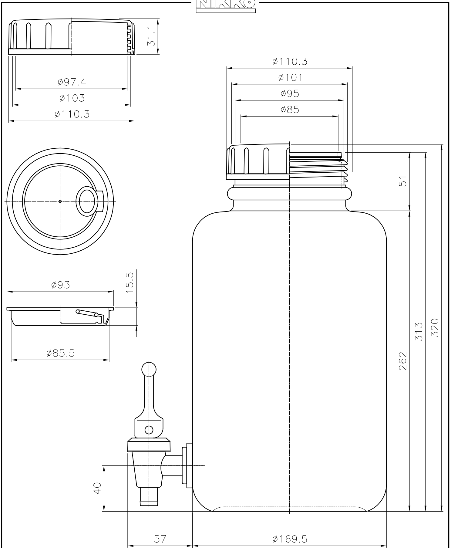
参考図面
