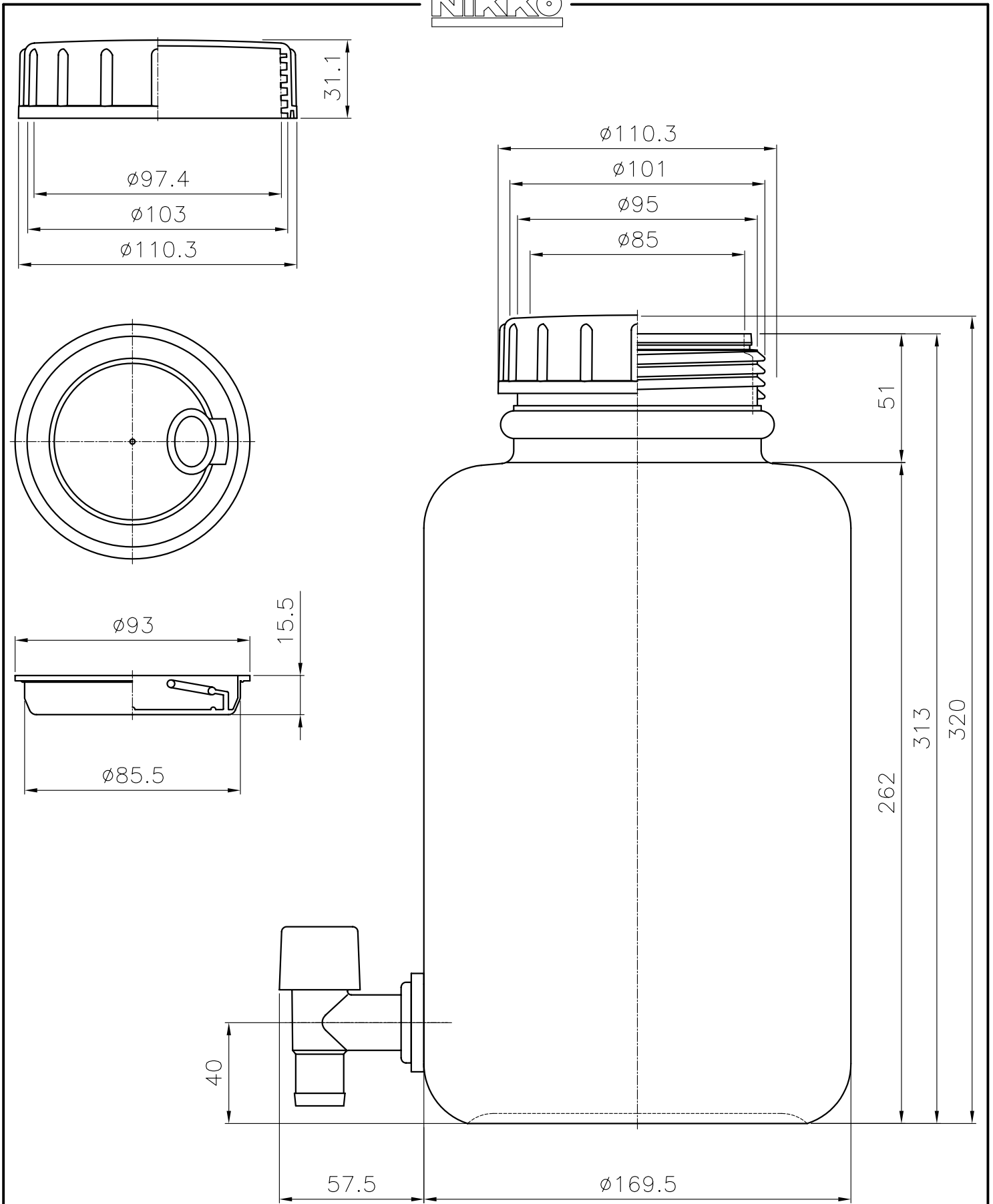
参考図面
