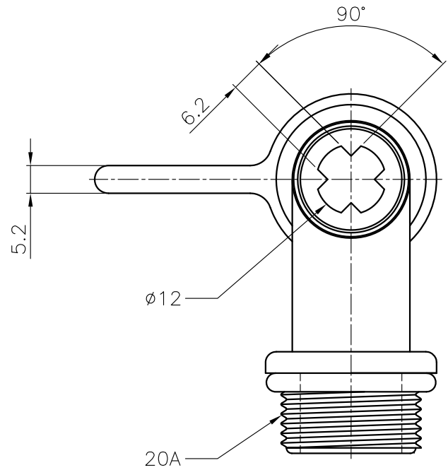
参考図面
