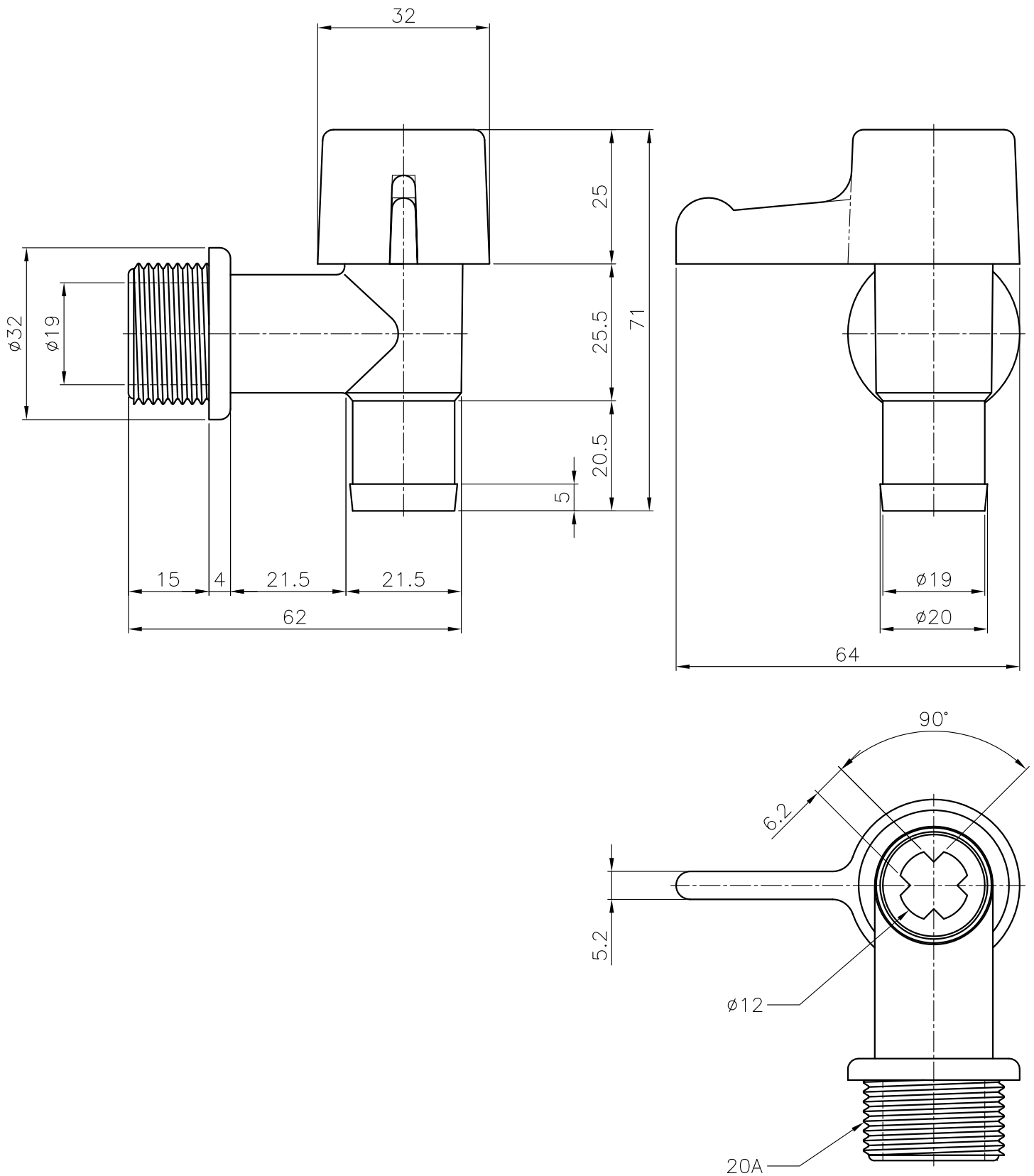
参考図面
